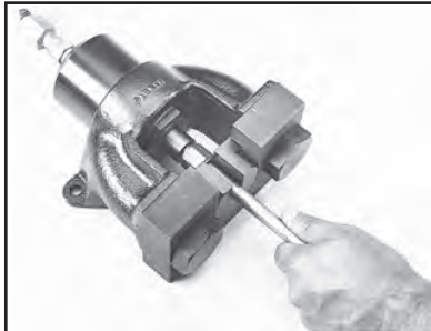
Fig. R36 – Hyferset tool
